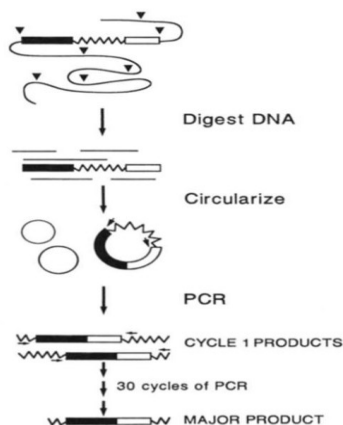
Slika 3. Shematski prikaz inverznog PCR-a
