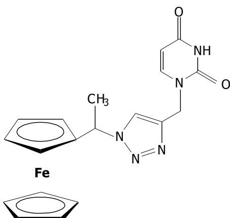
Slika 1. 1-[4-(1-Feroceniletil-1H-1,2,3-triazol-1-il)metil]uracil
