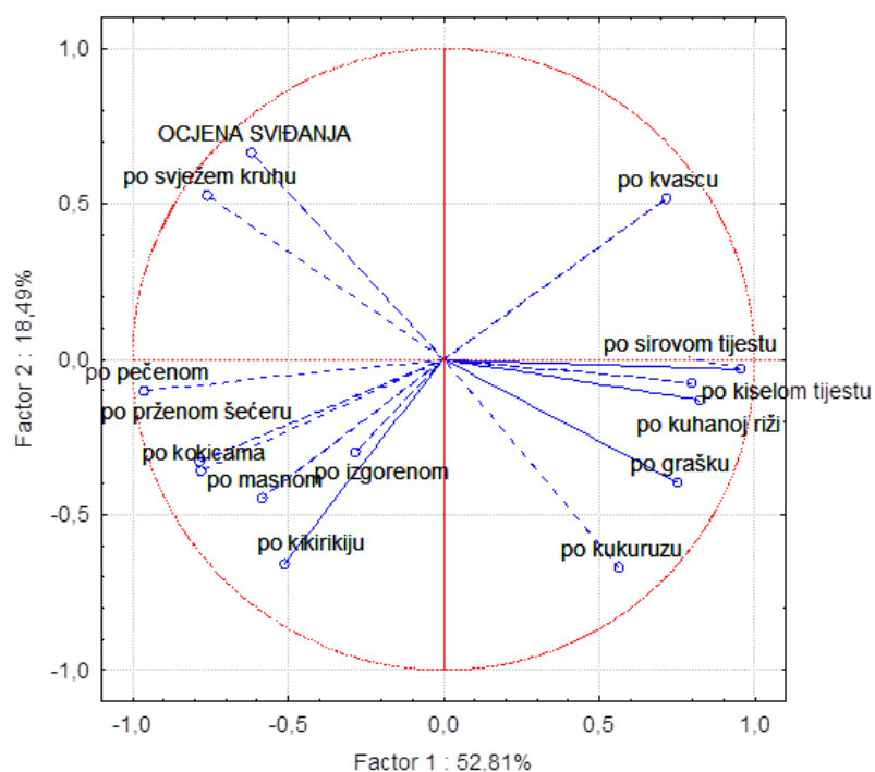
Slika 16. Faktorsko opterećenje (engl. loadings ) za prve dvije glavne komponente izračunato PCA analizom mirisnih atributa kore i sredine kruha
