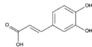
Kava kiselina
