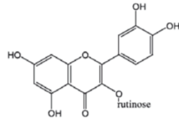
Rutin
