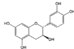
(+)-Katehin
