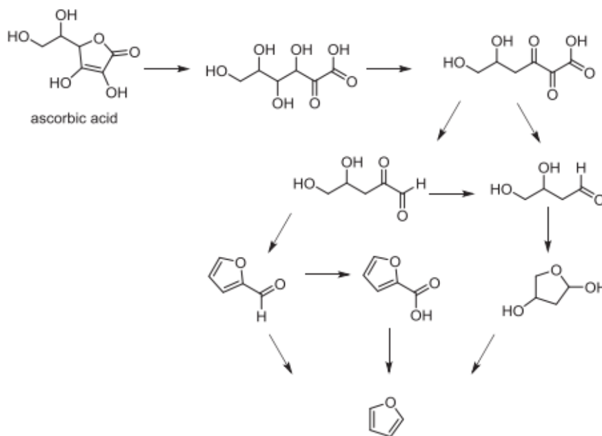
Slika 5. Shematski prikaz reakcija dobivanja furana iz askorbinske kiseline (Limacher et al., 2007)
