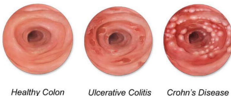
Slika 5. Razlike između izgleda zdravih crijeva, crijeva s ulceroznim kolitisom i crijeva kod Crohnove bolesti [51].
