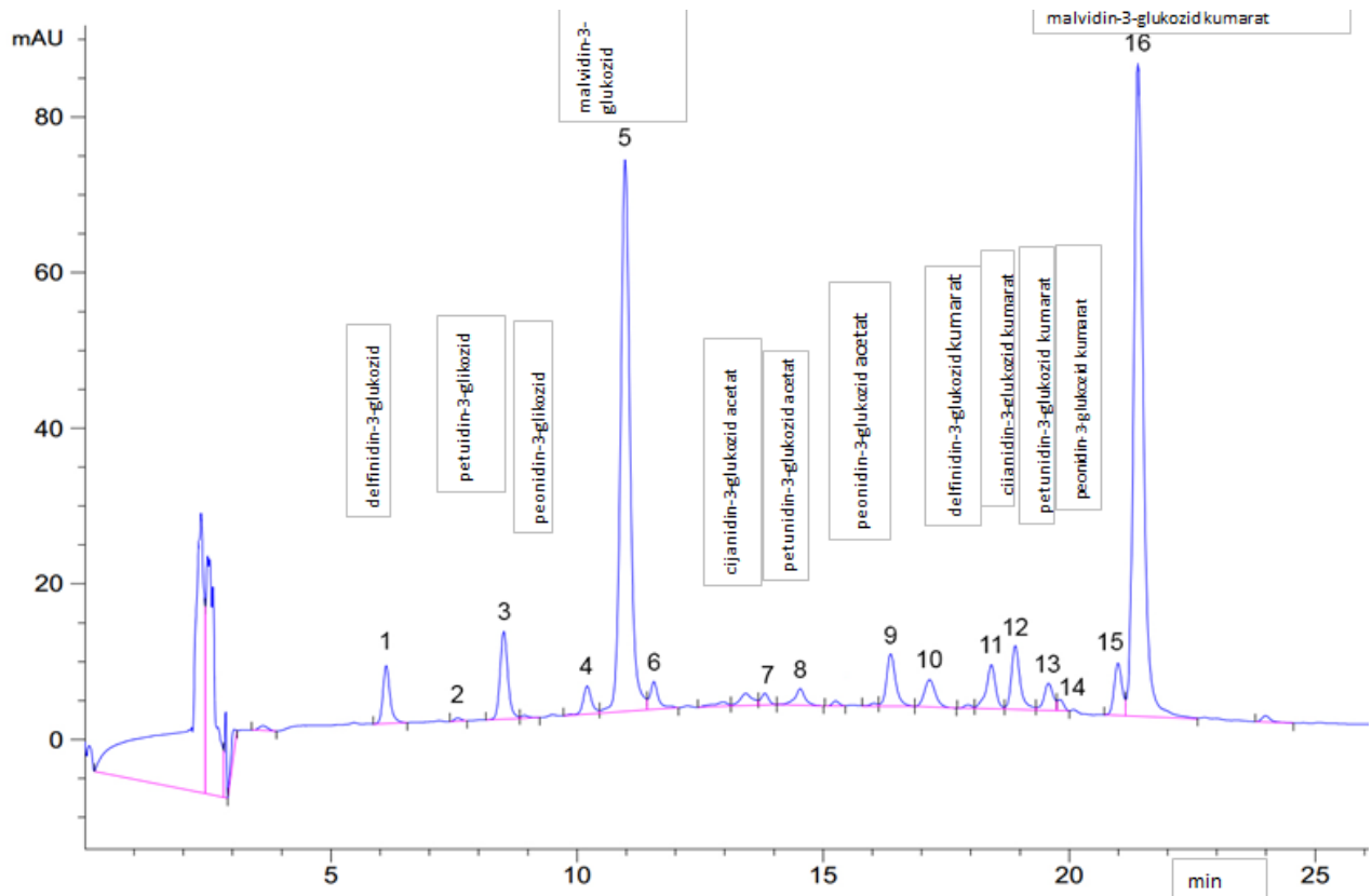
Slika 6. Tipičan kromatogram ekstrakta antocijana pokožice grožđa sa otapalom betain: limunska kiselina*
