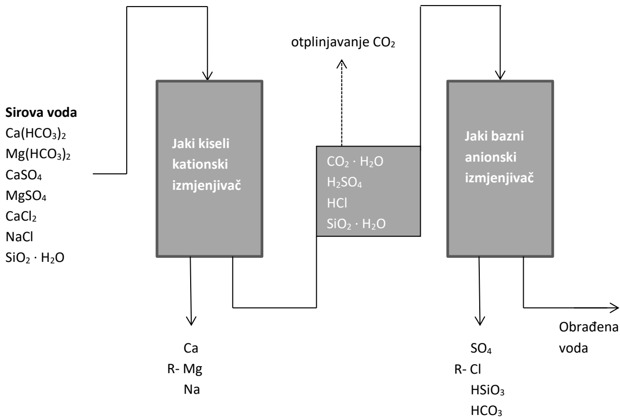
Slika 4 Ionski izmjenjivač
