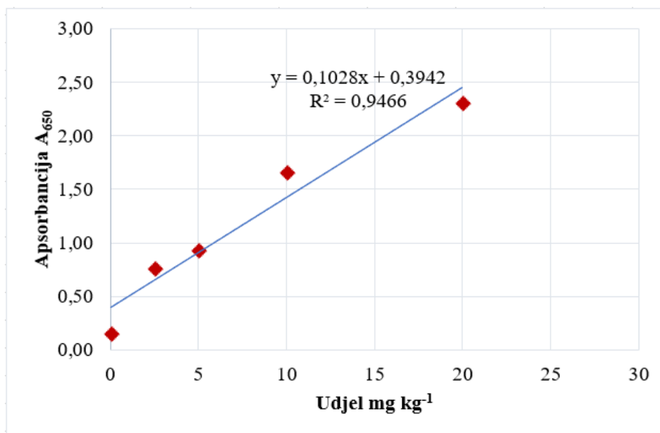
Slika 20. Baždarna krivulja standardnih otopina alergena lješnjaka ( RIDASCREEN® FAST Hazelnut ELISA test)
