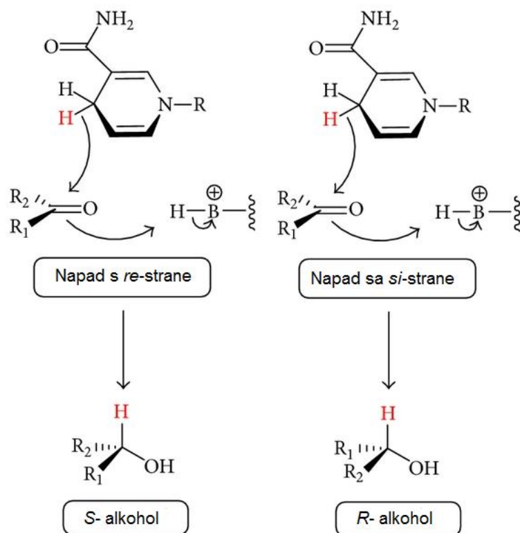
Slika 2. Primjer asimetrične redukcije prokiralnog ketona prema Prelogovom pravilu (Nguyen i sur., 2014)
