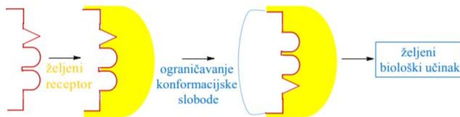
Slika 1. Ograničavanje konformacijske slobode i „zaključavanje“ bioaktivne konformacije (Barišić, 2018).
