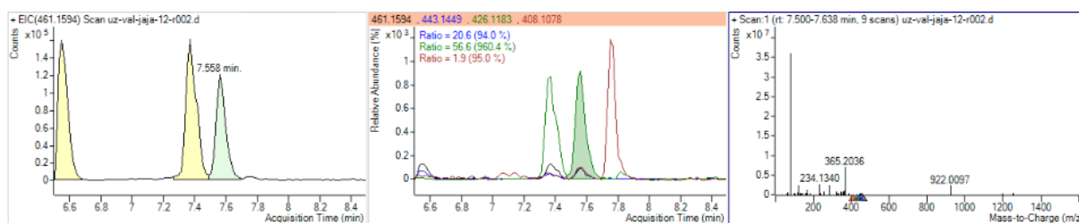
Slika 26. Kromatogrami produkata iona oksitetraciklina dobivenih na UHPLC/Q-TOF-MS uređaju: a) standard (L3 koncentracijska razina), b) negativni kontrolni uzorak (engl. Matrix blank ), c) obogaćeni uzorak (koncentracijska razina M3)
