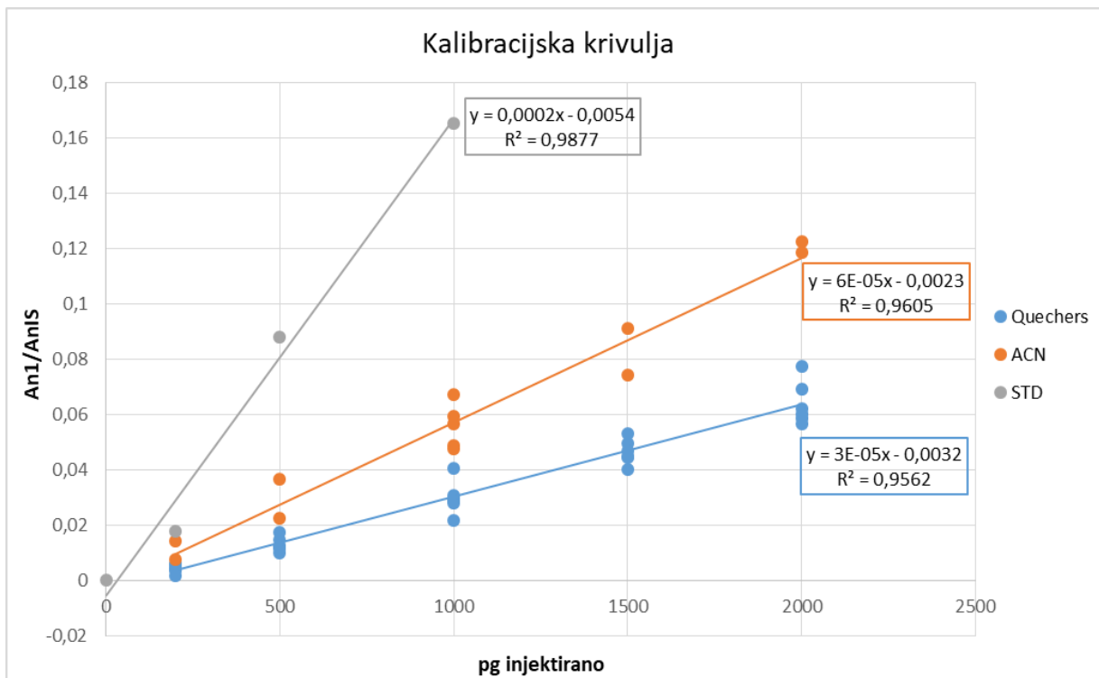
Slika 33. Usporedba standardne (STD) i matrics (Quechers, ACN) kalibracijske krivulje za oksitetraciklin na LC-MS/MS uređaju
