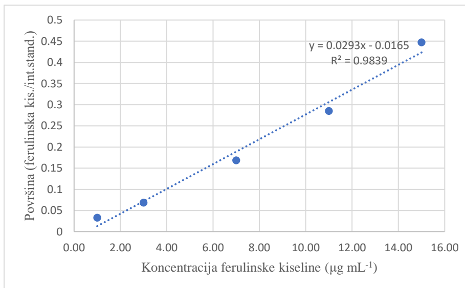
Slika 6. Baždarna krivulja za ferulinsku kiselinu s pripadajućom jednačicom
