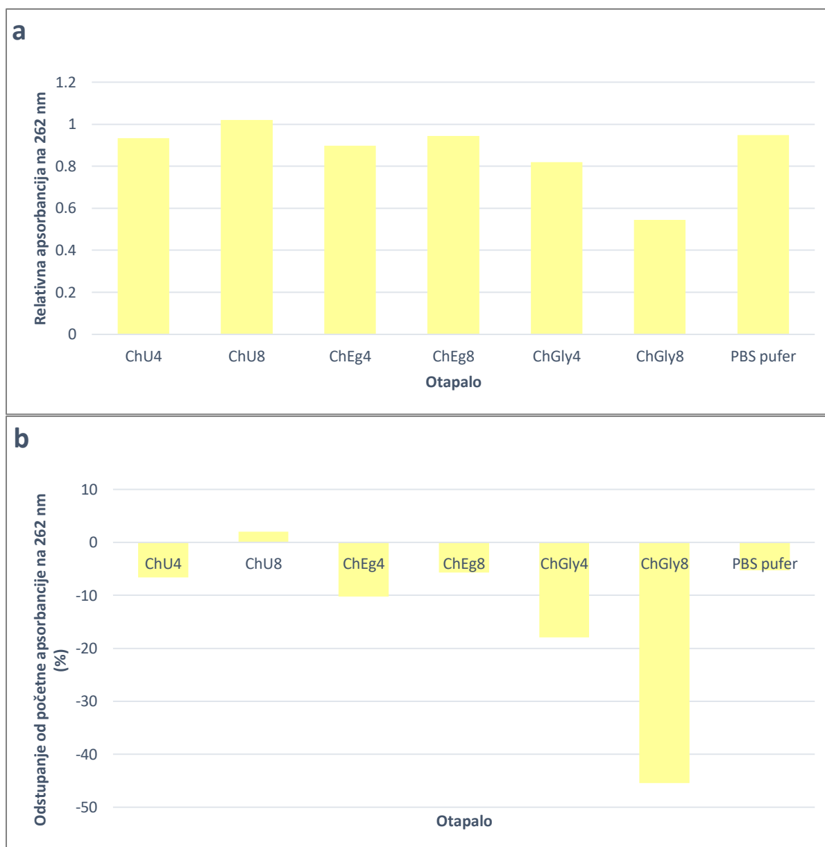
Slika 14. a) Relativna apsorbancija na 262 nm nakon 15 dana inkubacije NAD + u različitim otapalima pri 4 °C, b) Odstupanje (%) od početne apsorbancije na 262 nm nakon 15 dana inkubacije NAD + u različitim otapalima pri 4 °C. Rezultati su prikazani kao srednja vrijednost (n=2).
