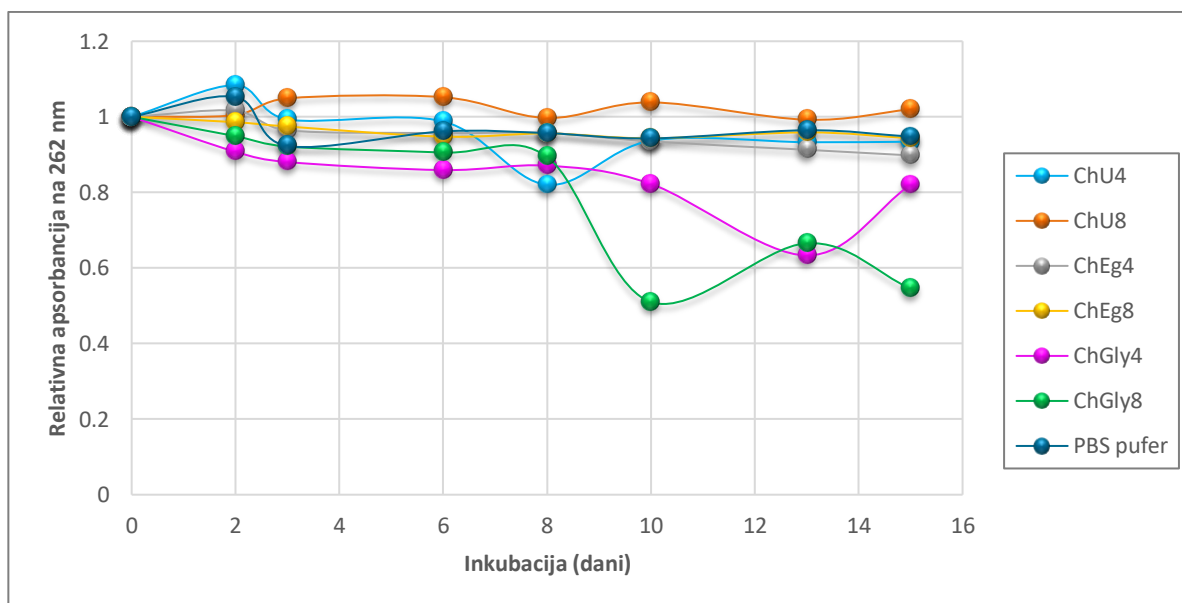
Slika 13. Relativna apsorbancija na 262 nm tijekom 15 dana inkubacije NAD + u različitim otapalima pri 4 °C. Rezultati su prikazani kao srednja vrijednost (n=2).
