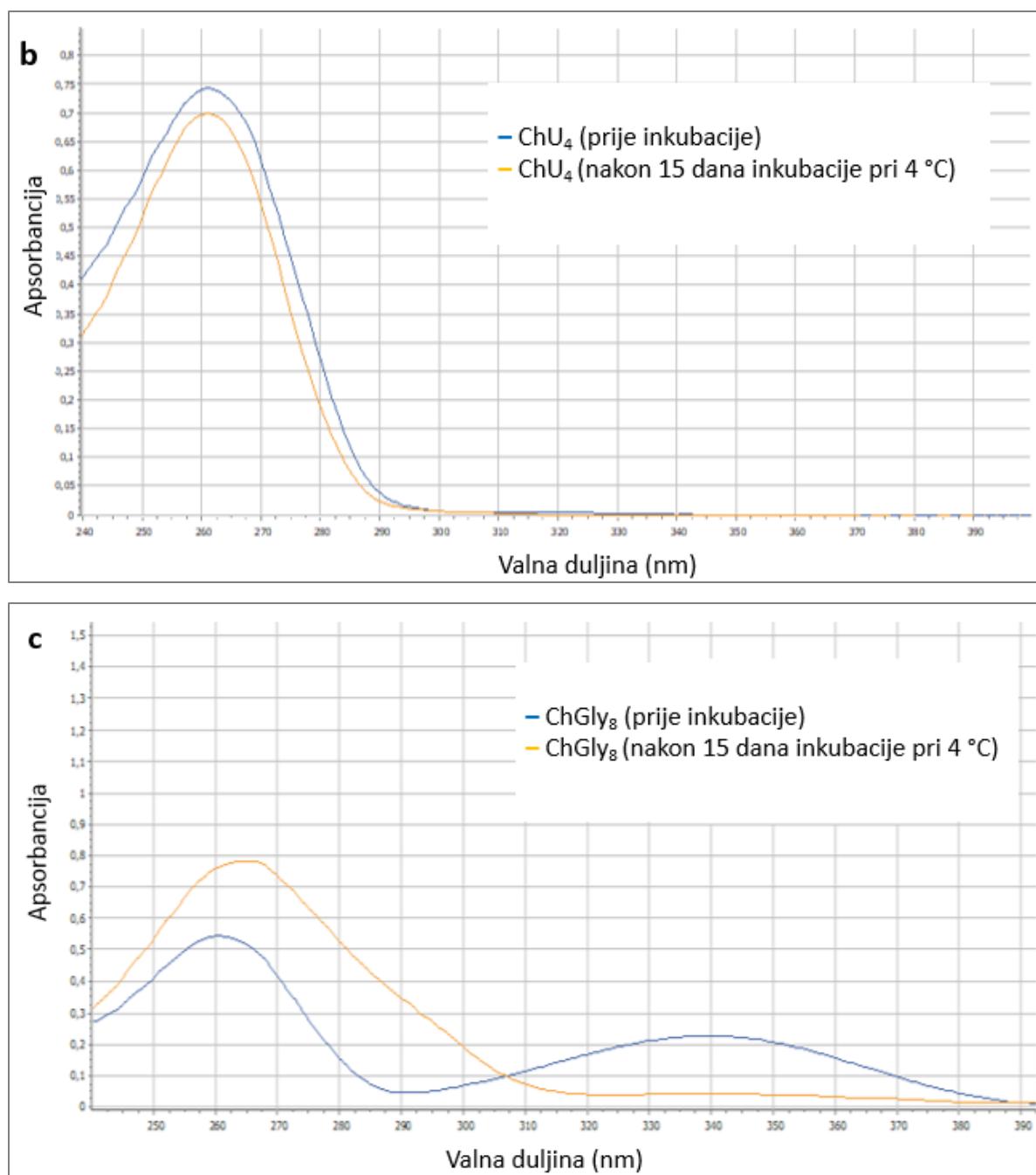
Slika 15. Promjene u apsorpcijskim spektrima koenzima a) NADH nakon 15 dana inkubacije u ChU 4 pri 4°C, b) NAD + nakon 15 dana inkubacije u ChU 4 pri 4°C, c) NADH nakon 15 dana inkubacije u ChGly 8 pri 4°C.
