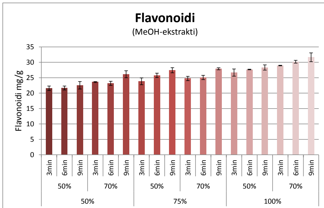
Slika 15. Rezultati spektrofotometrijskog određivanja ukupnih flavonoida u cvijetu trnina ( \text{mg g}^{-1} ) dobivenih metodom ekstrakcije potpomognute ultrazvukom primjenom 50 % i 70% vodenih otopina metanola u vremenu trajanja ekstrakcije 3, 6 i 9 minuta pri amplitudama od 50%, 75% i 100%. Rezultati su prikazani kao srednja vrijednost dvaju paralelnih određivanja \pm SD.
