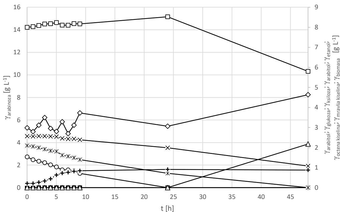
Slika 21. Uzgoj kvasca Spathaspora arborarie CBS 11463 u bioreaktoru na kiselinom hidrolizatu izluženih repinih reznaca (—□—arabinoza, —○— glukoza, —×— ksiloza —△— arabitol, —◇— biomasa, —+— mrvlja kiselina, —*— octena kiselina, —■— etanol)
