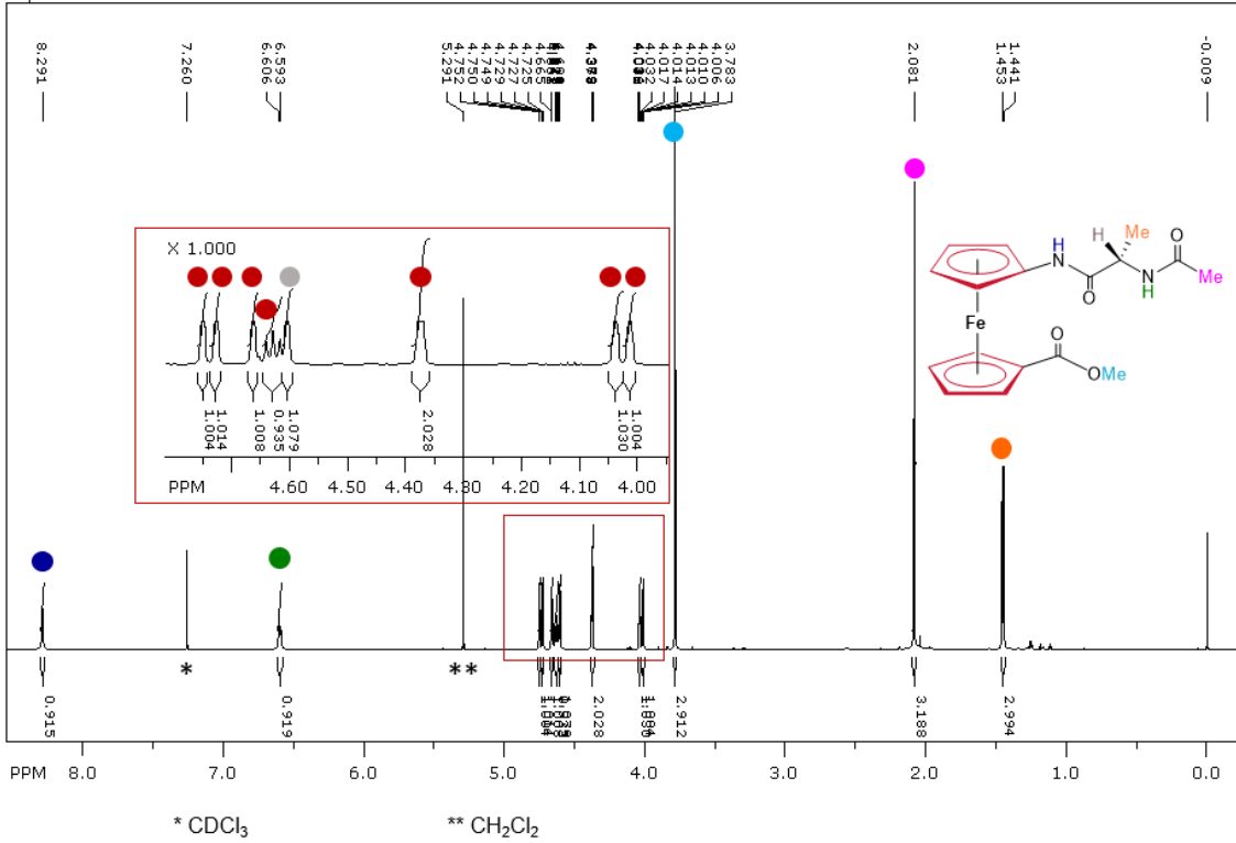
Slika 9. ^1\text{H} NMR-spektar dipeptida Ac-L-Ala-NH-Fn-CO-OMe (4).
