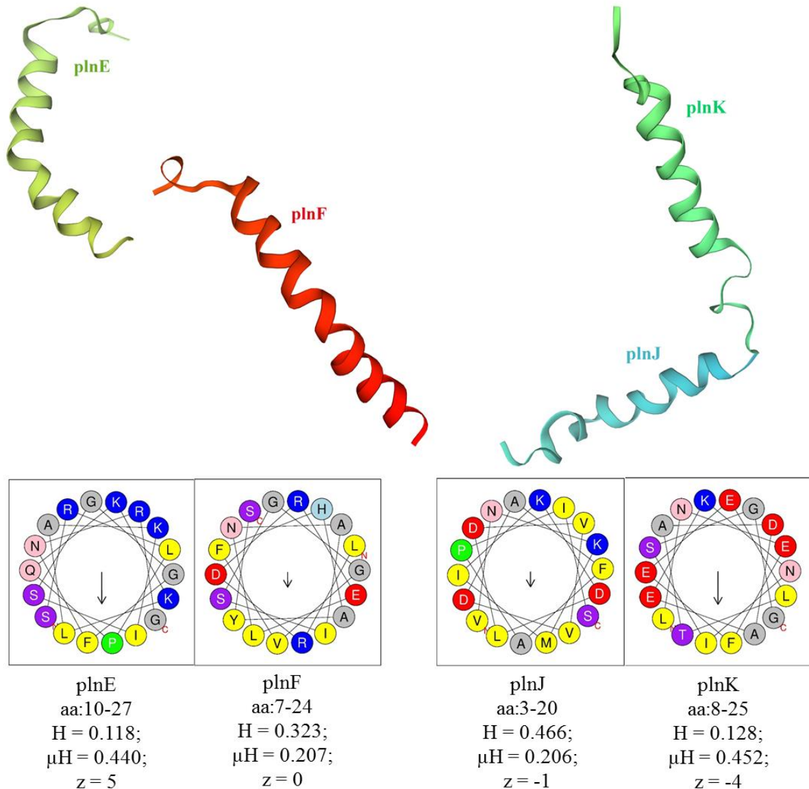
Slika 12. Trodimenzionalna struktura PlnJK i PlnEF soja L. plantarum D13, predviđena je modeliranjem pomoću metode prepoznavanja sličnosti primjenom SWISS-MODEL-a i prikaz svojstava \alpha -uzvojnica analiziranih primjenom HeliQuest servera. aa –aminokiseline); žuta – hidrofobne aa; ljubičasta – serinske i treoninske aa; tamno plava – bazične aa; crvena – kisele aa; roza – aparaginske i glutaminske aa; siva – alaninske i glicinske aa; svijetlo plava – histidinske aa; zelena – prolinske aa; H – hidrofobnost; \mu H – hidrofobni moment. Neto naboj (z) određen je pri pH = 7,4, pod pretpostavkom da je aminokiselina histidin neutralna i da su N-terminalna amino skupina i C-terminalna karboksilna skupina sekvence nisu nabijene
