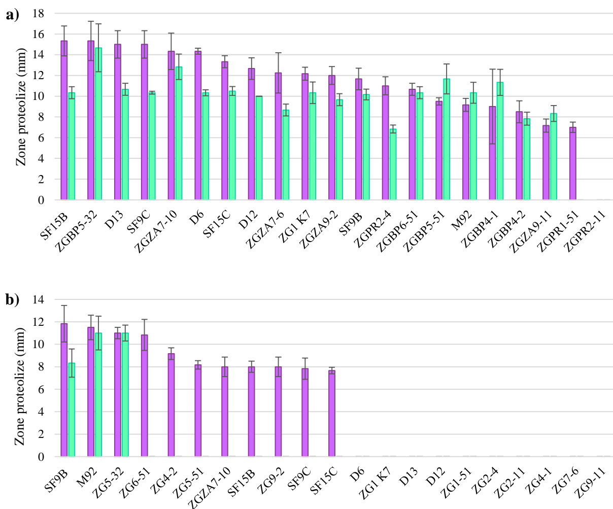
Slika 24. Kazeinolitička aktivnost ispitana je u uzorcima supernatanta prekonoćne kulture (■) i koncentrirane biomase (■) sojeva poraslih u a) optimalnom mediju i b) obranom mlijeku
