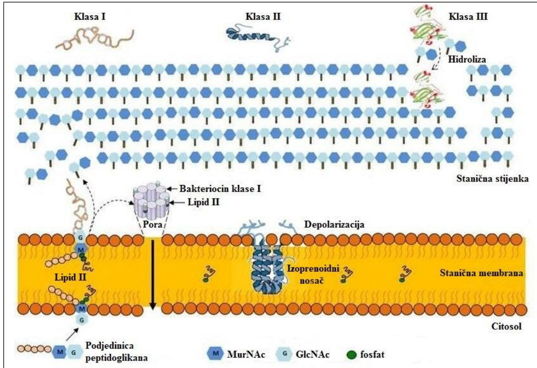
Slika 4. Mehanizam djelovanja bakteriocina bakterija mliječne kiseline (Alvarez-Cisneros i sur., 2011; uz dopuštenje autora)
