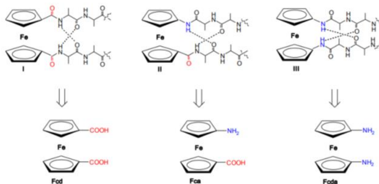
Slika 4. Ferocenski peptidi I-III izvedeni iz Fcd, Fca, Fda (isprekidane linije označavaju IHB) (prema Kovačević, 2014)
