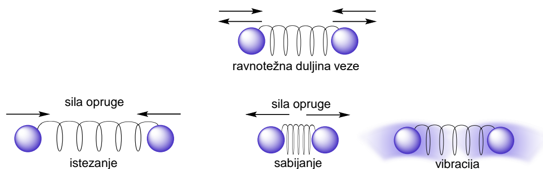
Slika 62. Molekulske vibracije.
