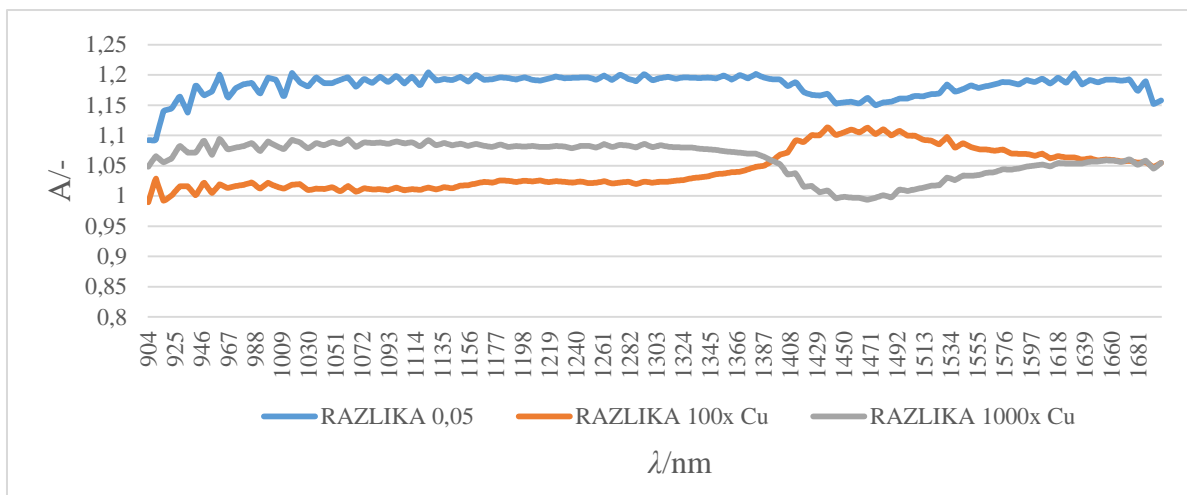
Slika 28. Prikaz NIR spektara kontaminiranih jabuka (Cuprablau Z 35 WG) nakon što su se srednje vrijednosti njihovih apsorbancija umanjile za srednje vrijednosti apsorbancija netretiranih jabuka za prvi dan (srednje vrijednosti apsorbancija originalnih otopina (RAZLIKA 0,05 Cu) i otopina koje su sto (RAZLIKA 100X Cu) i tisuću puta (RAZLIKA 1000X Cu) razrjeđenije od originalne, umanjene za srednje vrijednosti apsorbancija netretiranih jabuka)
