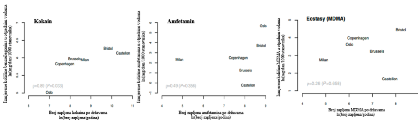
Slika 3. Broj zapljena kokaina, amfetamina i ecstasyja, te količine benzoilegonina, amfetamina i MDMA određene u otpadnim vodama u Oslu, Copenhagenu, Bristolu, Castellonu, Milanu i Bruxellesu ( prema Baz-Lomba i sur., 2016)
