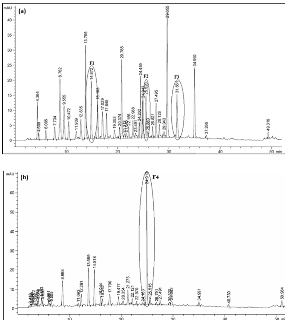
Slika 21. Kromatogrami (snimljeni na 320 nm) ekstrakta dobičice (uzorak D5) dobiveni: a) ekstrakcijom potpomognutom mikrovalovima i b) ekstrakcijom subkritičnom vodom; i izdvojene frakcije F1, F2, F3 i F4
