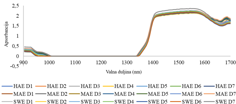
Slika 30. NIR spektri ekstrakata dobričice
