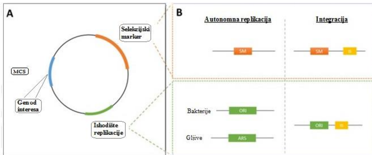
Slika 1. Shematski prikaz ekspresijskog vektora. A. Ekspresijski vektor sadrži ishodište replikacije (ORI), višestruko mjesto kloniranja (MCS) u koje je integriran gen od interesa i slijedi seleksijski marker (SM). B. Episomalni i integrativni plazmid. ARS, autonomna replikacijska sekvenca; IS, integracijsko mjesto (Deckers i sur., 2020)
