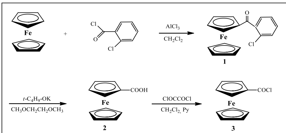
Shema 2. Priprava ferocenkarkobsilne kiseline (2) i ferocenoil klorida (3)
