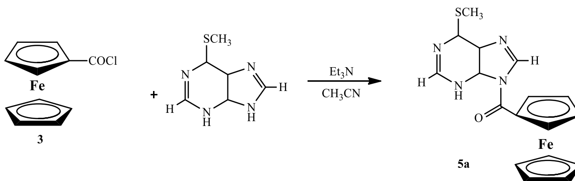
Shema 7. Shema priprave N 9-ferocenoil-6-metilmercaptapurina ( 5a )
