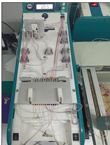
Slika 10. Analitička jedinica sa sustavom cijevi u kojima se odvija kontinuirani protok ( vlastita fotografija )
