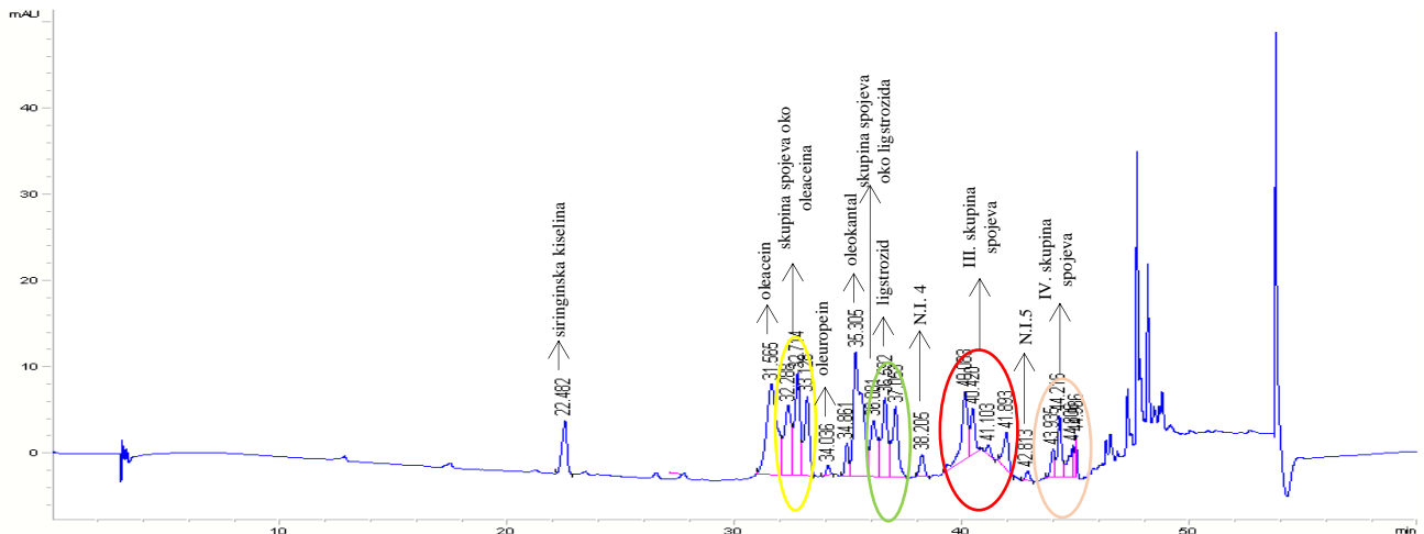
Slika 3. Kromatogram fenolnih spojeva djevičanskog maslinovog ulja sorte Levantinka
