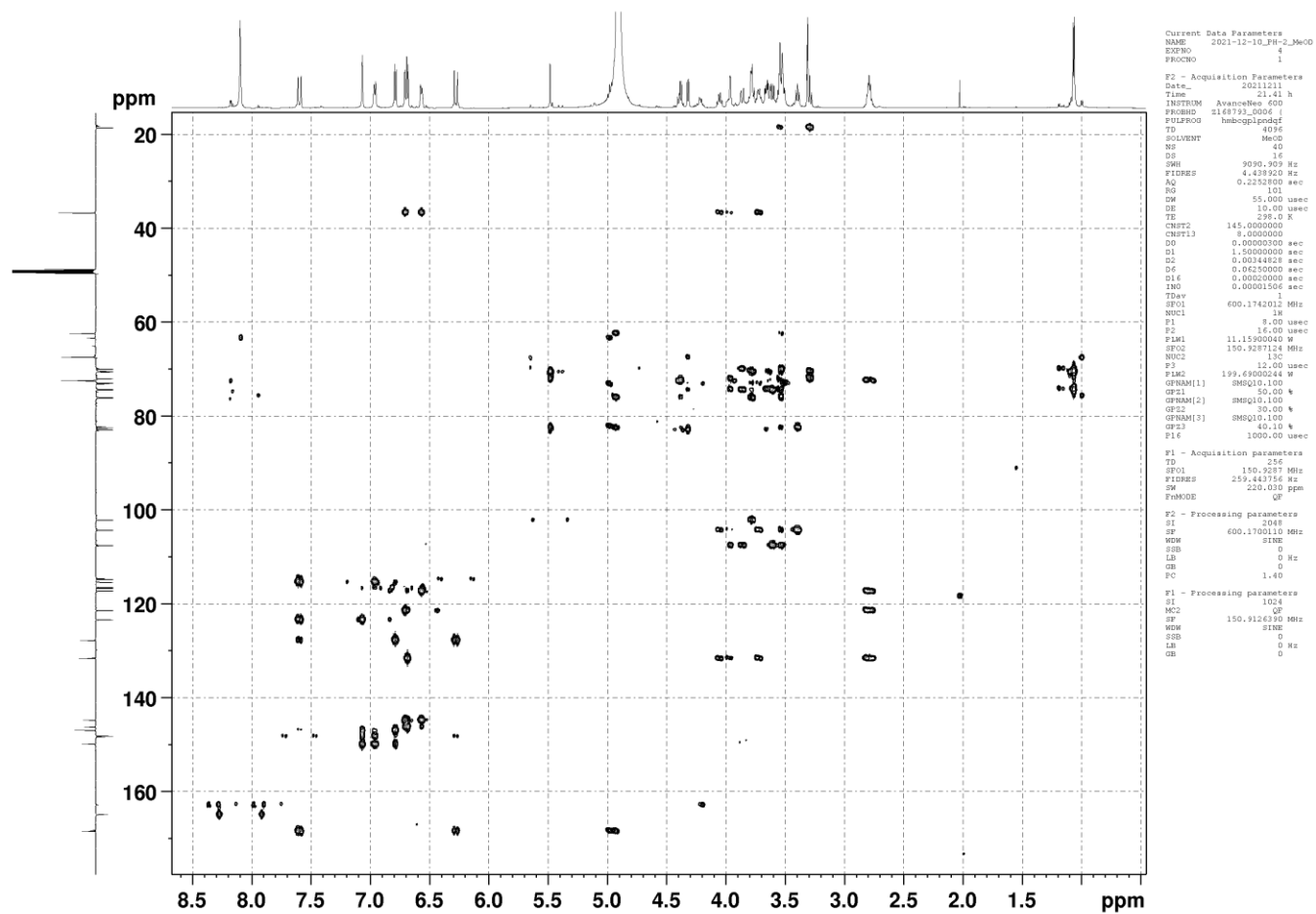
Prilog 22. Spektar ^1\text{H} - ^{13}\text{C} HMBC polifenolne frakcije stahizoida A u metanolu- \text{d}_4 pri 25 °C
