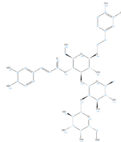
Prilog 12. Spektar 1 H polifenolne frakcije teupolizida u metanolu-d 4 pri 25 °C
