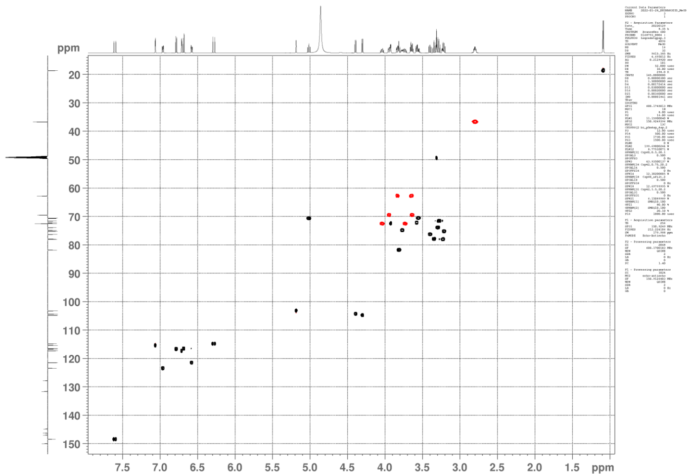
Prilog 4. Spektar ^1\text{H} - ^{13}\text{C} HSQC spoja chinakozida u metanolu- \text{d}_4 pri 25 °C
