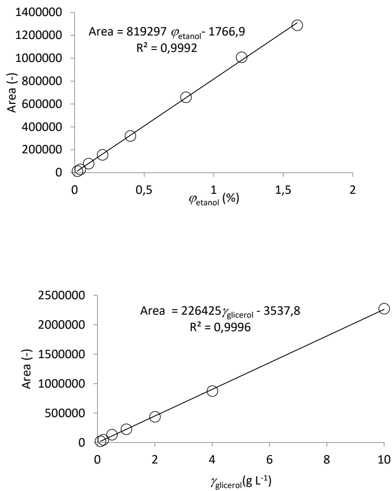
Slika 15 Baždarni pravci za određivanje ugljikohidrata, alkohola i kiselina prisutnih u pivu HPLC metodom.
