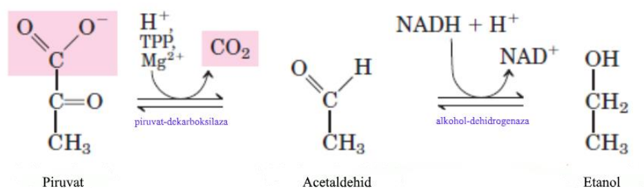
Slika 3. Biokemijska reakcija nastajanja etanola (Anonymus 2, 2017)
