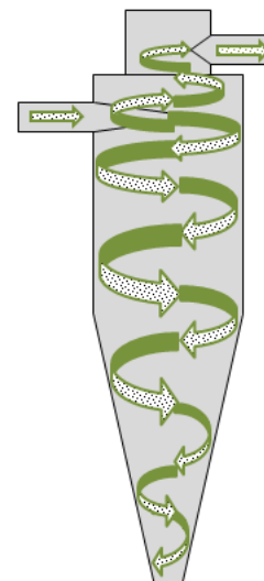
Slika 7. Kretanje čestice praha i izlaznog zraka u ciklonu (prema Anonymous, 2017)
