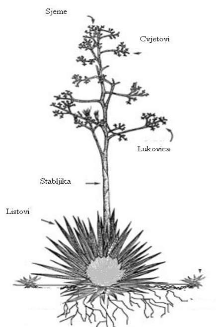
Slika 1. Struktura Agave tequilana Weber var. azul
