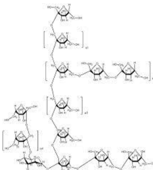
Slika 12. Miješani fruktni povezani \beta -(2-1) i \beta -(2-6) vezama između molekula fruktoze
