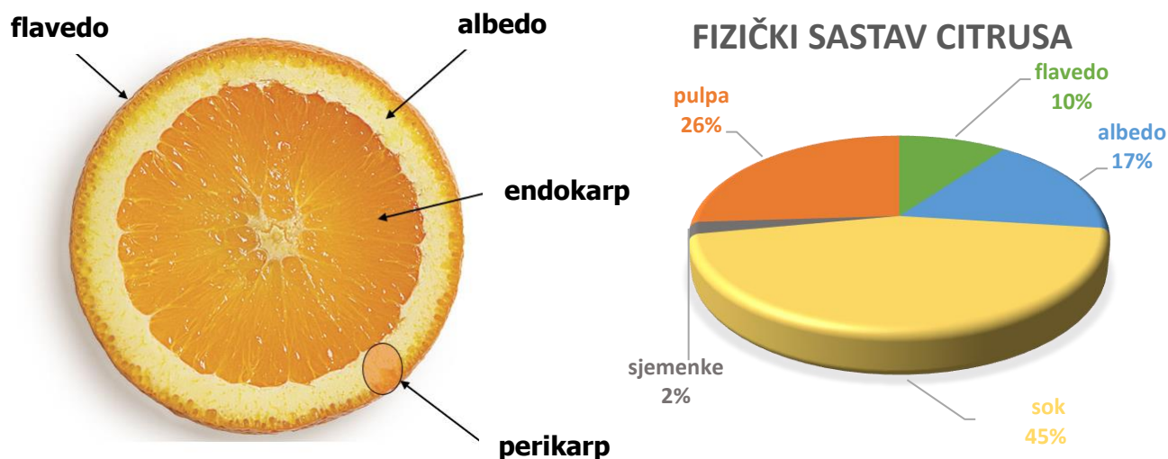
Slika 2. Struktura citrusa (Mahato i sur.,2018).
