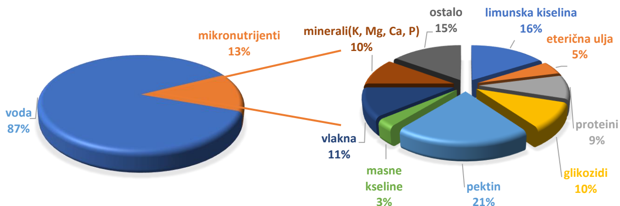
Slika 3. Kemijski sastav citrusa (Mahato i sur., 2018).
