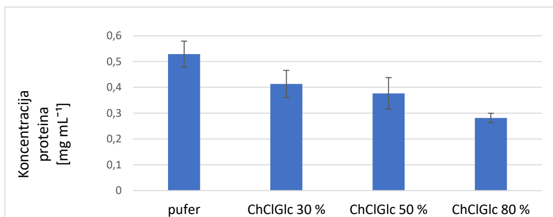
Slika 11. Koncentracija proteina u ekstraktima kore naranče*.
