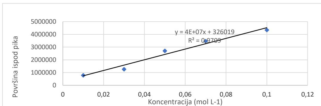
Slika 14: Baždarni dijagram za određivanje koncentracije (R,S)-1-feniletil-acetata.
