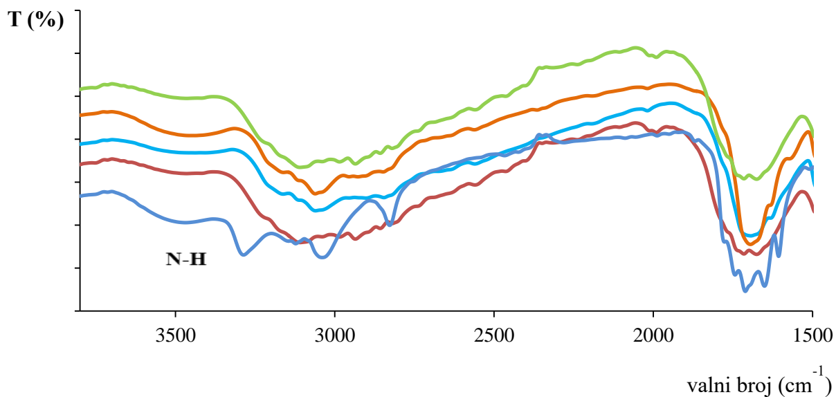
Slika 31. Dio IR spektra spojeva 12a-e
