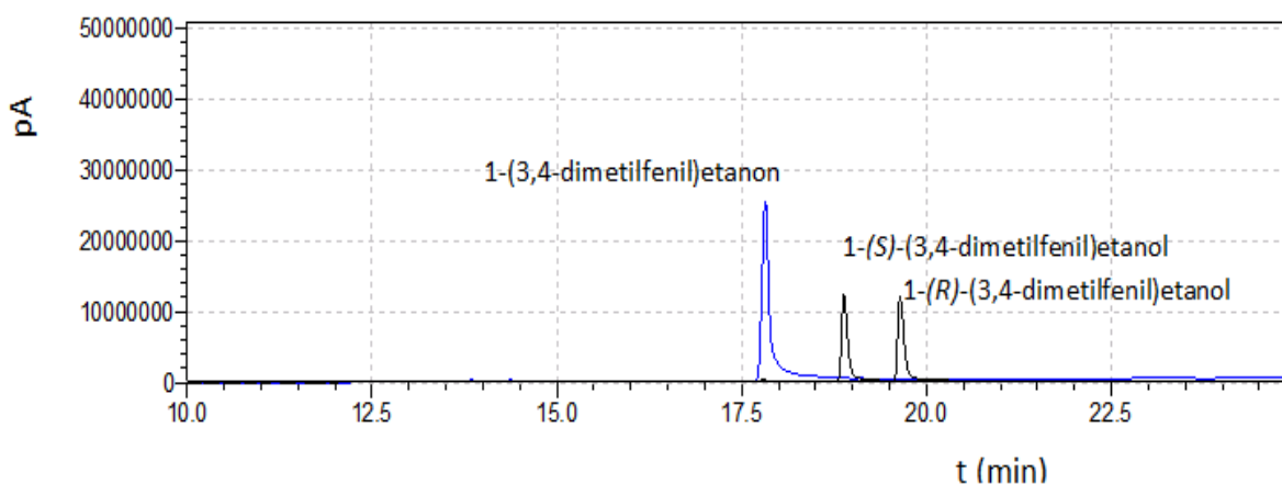
Slika 10. Tipičan GC kromatogram analize reakcijske smjese enantioselectivne redukcije 1-(3,4-dimetilfenil)etanona
