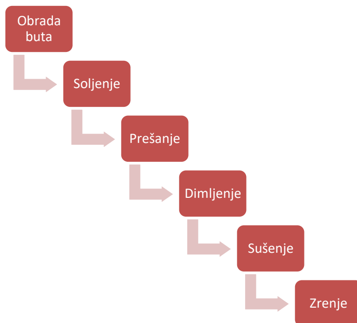
Slika 2. Tehnološki postupak proizvodnje dalmatinskog pršuta
