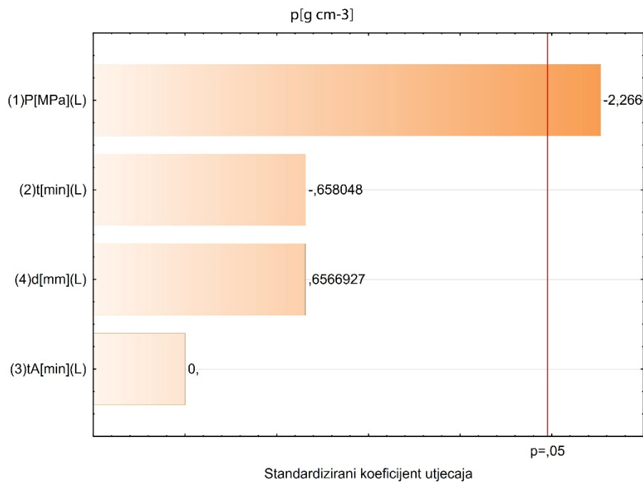
Slika 22. Pareto dijagram – utjecaj visokog hidrostatskog tlaka i vremena obrade na gustoću [g cm -3 ], smoothieja S_{0,5} i S_{0,3} izraženog preko standardiziranog koeficijenta utjecaja ( \beta )
