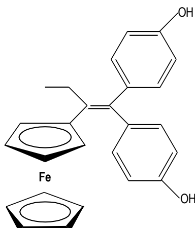
Slika 10. 1,1-di-(4'-hidroksifenil)-2-ferocenil-but-1-en
