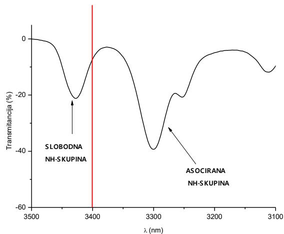
Slika 26. Prikaz područja istežnih frekvencija NH-skupina
