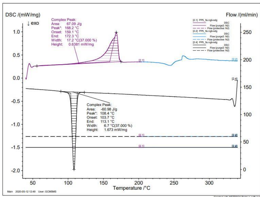
Slika 10. Prikaz ovisnosti protoka topline o temperaturi za PP/Ac/PVDC ambalažu tretiranu na udaljenosti 7,23 cm i 5 sekundi
