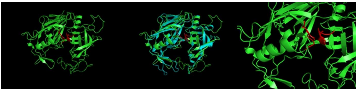
Slika 12. Model Yps6 (zeleno), preklopljen s predloškom 2h6s (plavo) i uvećano katalitičko mjesto. Katalitički aspartatni ostatci označeni su crvenom bojom.
