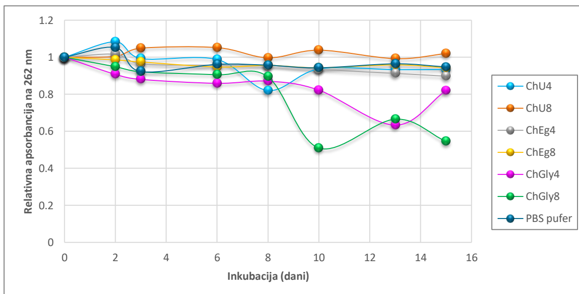
Slika 13. Relativna apsorbancija na 262 nm tijekom 15 dana inkubacije NAD + u različitim otapalima pri 4 °C. Rezultati su prikazani kao srednja vrijednost (n=2).
