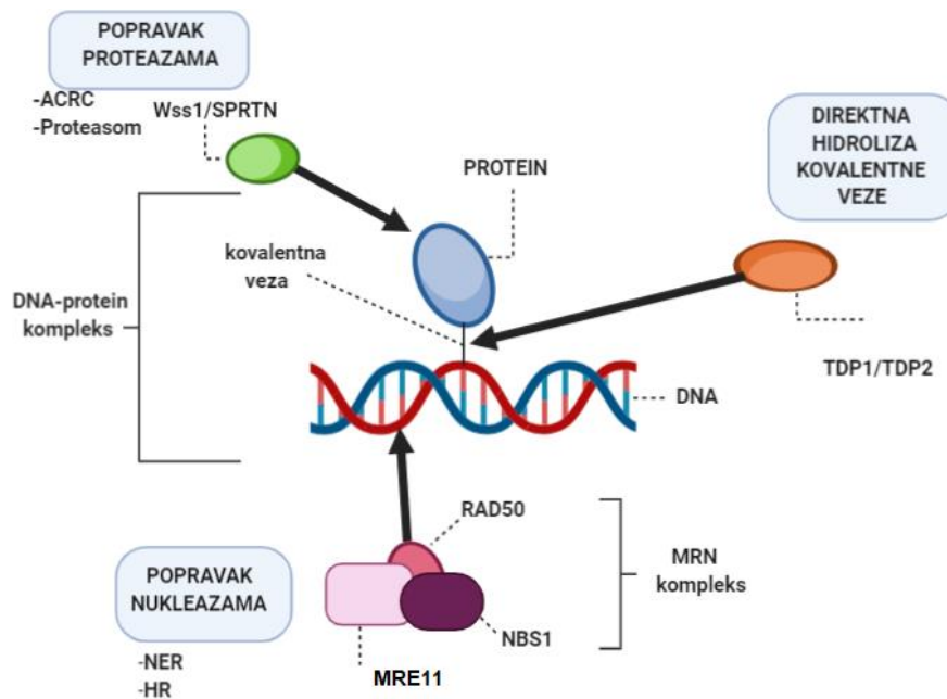
Slika 3. Tipovi DPC popravka (engl. DNA-protein crosslink repair ) ( Acrc - Acidic repeat containing protein , NER – Nucleotide Excision Repair (nukleotidni ekscizijski popravak), HR – Homologous Recombination (homologna rekombinacija), Tdp1/2 – tirozil-DNA fosfodiesteraza 1/2, MRN kompleks – Mre 11 , Nbs1 , Rad50 ) (20).
