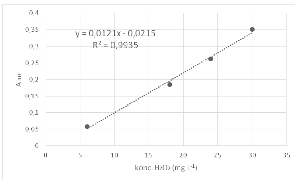
Slika 11. Baždarni dijagram ovisnosti apsorbancije o koncentraciji H 2 O 2
