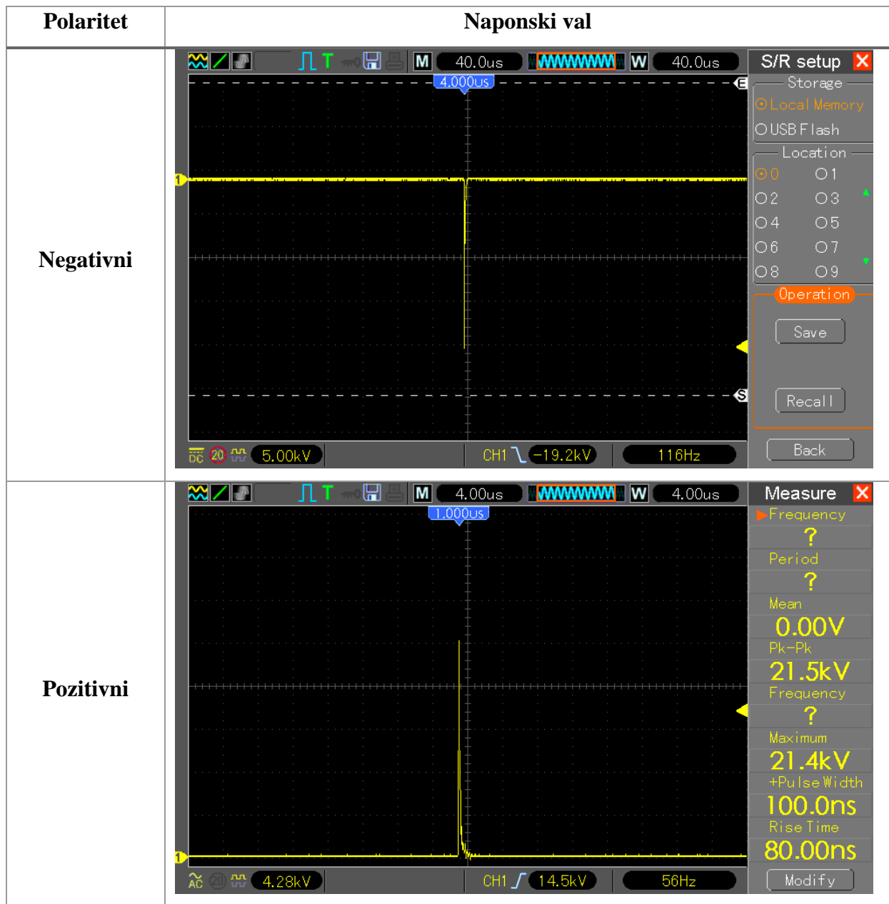
Tablica 10. Grafički prikaz naponskog vala tijekom tretmana plinskom plazmom
