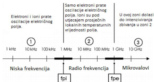
Slika 3. Primjer raspona varijacije za f_{pi} (ionsku frekvenciju) i f_{pe} (frekvencije elektrona) u hladnoj plazmi tj. svjetlećim izbojima (Tendero i sur., 2006)
