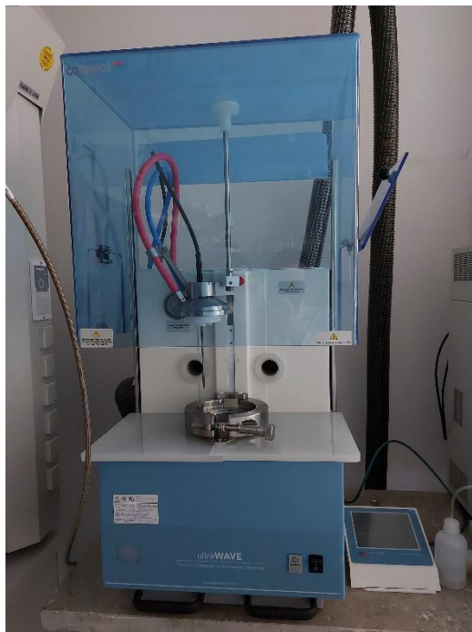
Slika 10. Mikrovalna pećnica korištena za razgradnju uzorka (Vlastita fotografija)
