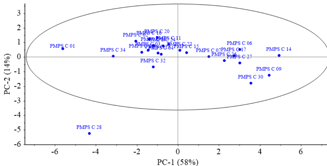
Slika 191. Raspodjela faktorskih bodova PC1 i PC2 matematički obrađenih (SNV i uklanjanje trenda polinomom 4. stupnja) Raman spektara PMPS C u spektralnom području \tilde{\nu} = 3500 - 100 \text{ cm}^{-1} sa Hotelling T 2 elipsom (interval pouznanosti 95 %) sa centrom modela u sjecištu dvaju pravaca (sivo).
