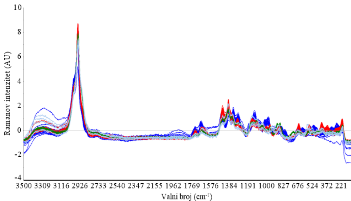
Slika 132. Raman spektri PMPS A (plavo), C (crveno), W135 (zeleno) i Y (sivo) matematički obrađeni standardnom normalnom varijatom (SNV) u spektralnom području \tilde{\nu} = 3500 - 100 \text{ cm}^{-1} .
