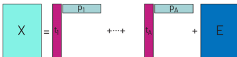
Slika 8. Razlaganje PC (prilagođeno iz Pomerantsev, 2014). X – inicijalna matrica; t_1 - t_A - projekcije uzoraka u novom koordinatnom sustavu; p_1 - p_A ; - projekcija varijabli u novom koordinatnom sustavu; E – matrica reziduala.
