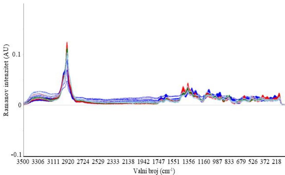
Slika 133. Raman spektri PMPS A (plavo), C (crveno), W135 (zeleno) i Y (sivo) matematički obrađeni jediničnom vektorskom normalizacijom u spektralnom području \tilde{\nu} = 3500 - 100 \text{ cm}^{-1} .
