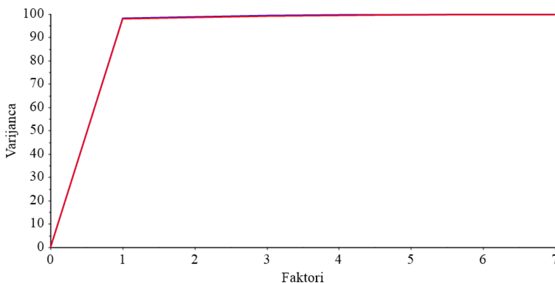
Slika 232. Kumulativna kalibracijska i validacijska varijanca za svaki PLS faktor. Kalibracija (plava linija), validacija (crvena linija).
