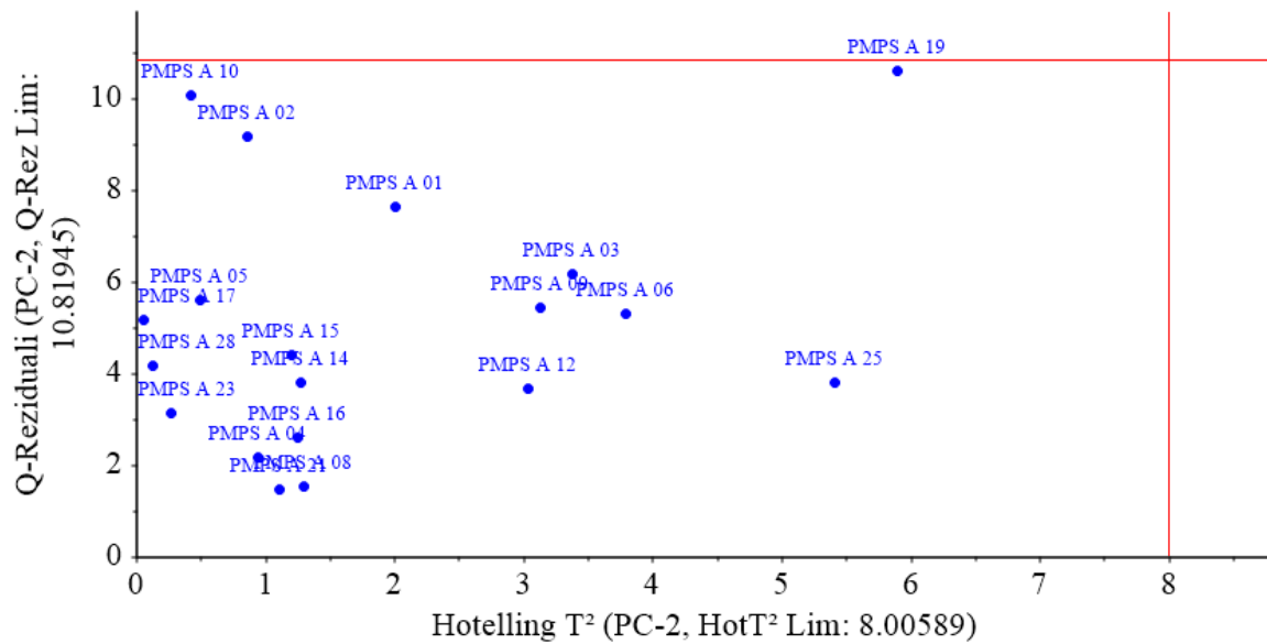
Slika 177. Hotelling T^2 statistika i Q-reziduali uzoraka PMPS A za PC2 s pripadajućim graničnim vrijednostima (okomita i vodoravna crvena linija).
