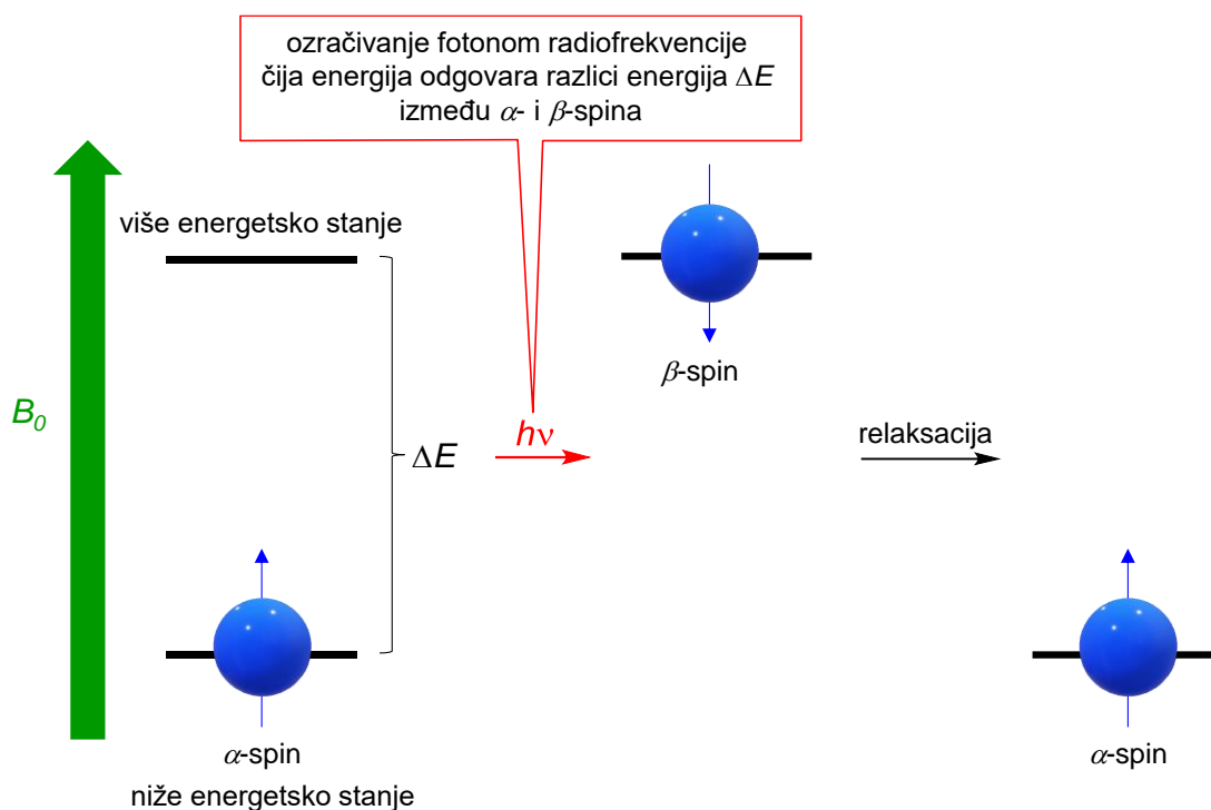
Slika 72. Rezonancija – izvrtnanje jezgre iz stanja \alpha -spina u \beta -spina i vraćanje u početno stabilnije \alpha -spinsko stanje.
