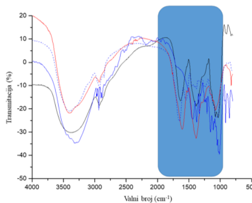
e) IR spektar ekstrakta dobričice (—); djelomično hidrolizirane guar gume (DHGG) (—); mucina (- - -); inkapsulata pripremljenog s DHGG i mucinom (—)
