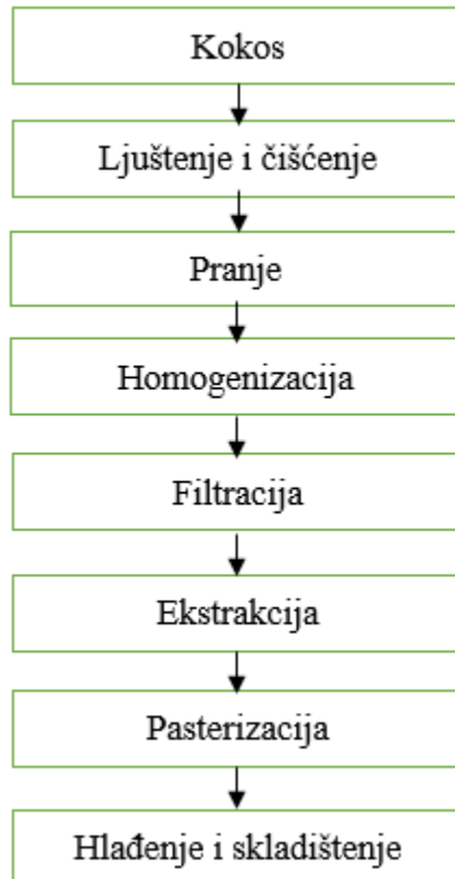
Slika 3. Shema tehnološkog procesa (prema Tulashie i sur., 2022)
