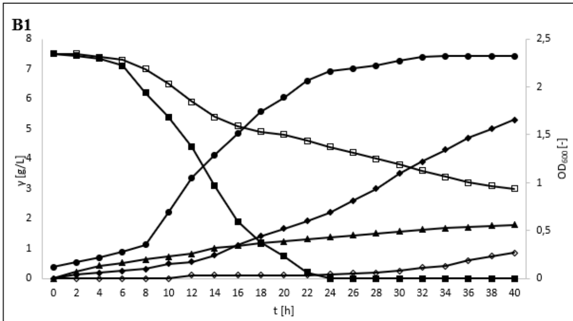
Slika 6. Ovisnost koncentracije supstrata, produkta i OD o vremenu tijekom uzgoja P. polymyxa DSM 742 na: B - kemijski definiranoj podlozi koja je sadržavala glukozu i ksilozu kao izvore dušika, B 1 – kemijski definiranoj podlozi B u koju je dodano i 4 g/L kvašćevog ekstrakta
