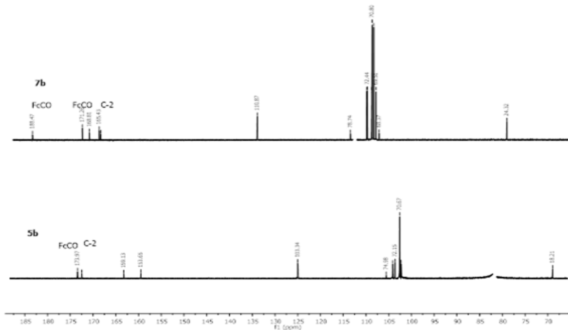
Slika 25. 13 C NMR spektar ferocenoil-6-metil-2-tiouracila ( 5b ) i S/N3 -bisferocenoil-6-metil-2-tiouracila ( 7b )
