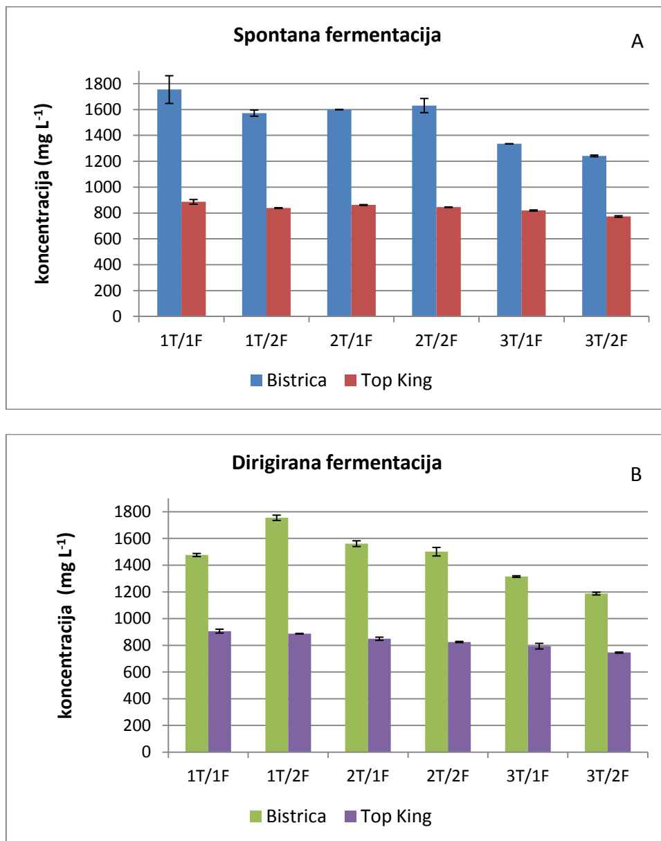
Slika 14. Usporedba koncentracija metanola u pojedinim frakcijama triju glavnih tokova destilata dobivenih destilacijom: A- spontano te B- dirigrano prefermentirane komine šljive Bistrice i Top King.
