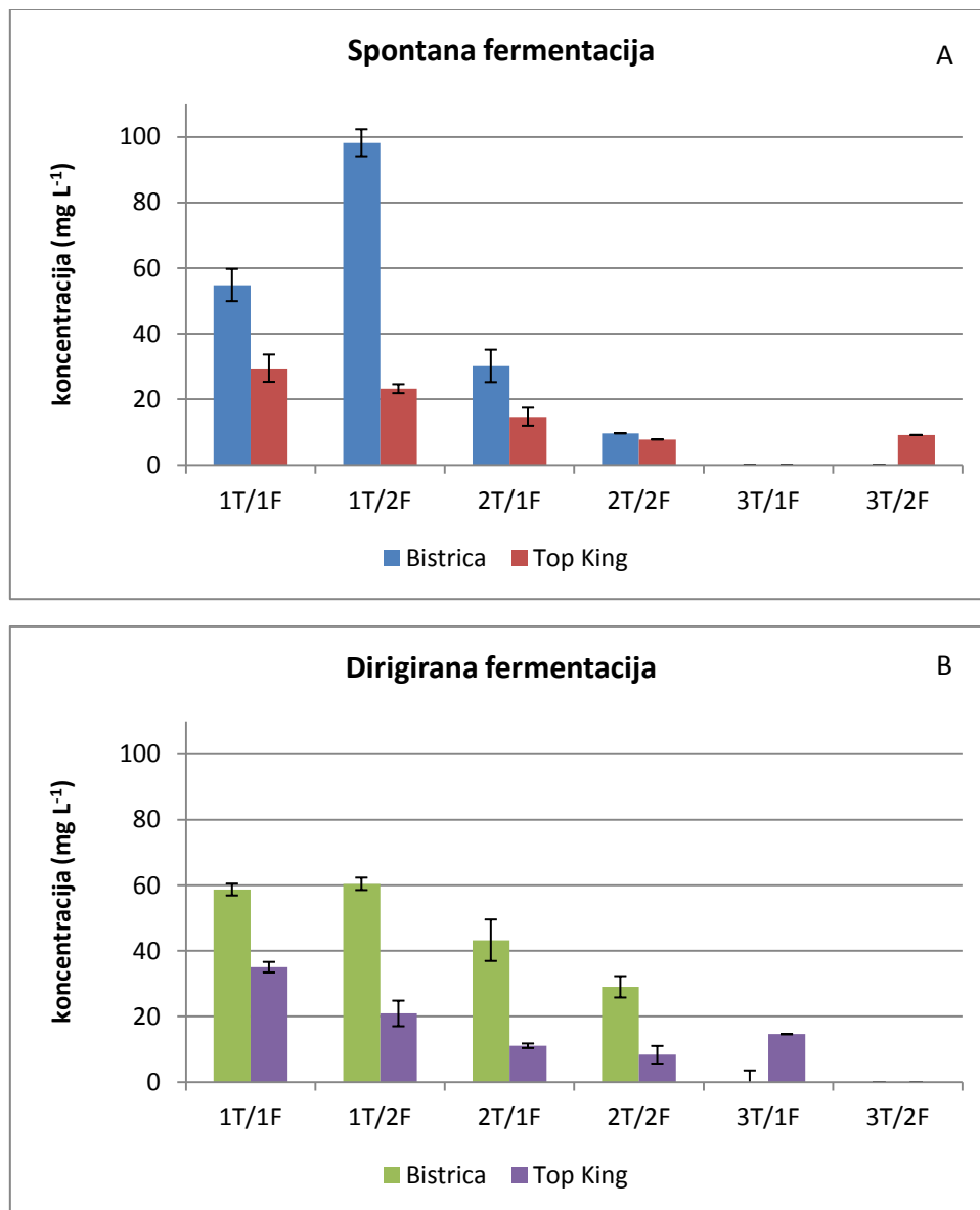
Slika 23. Usporedba koncentracija 2- feniletil acetata u pojedinim frakcijama triju glavnih tokova destilata dobivenih destilacijom: A- spontano te B- dirigrano prefermentirane komine šljive Bistrice i Top King.
