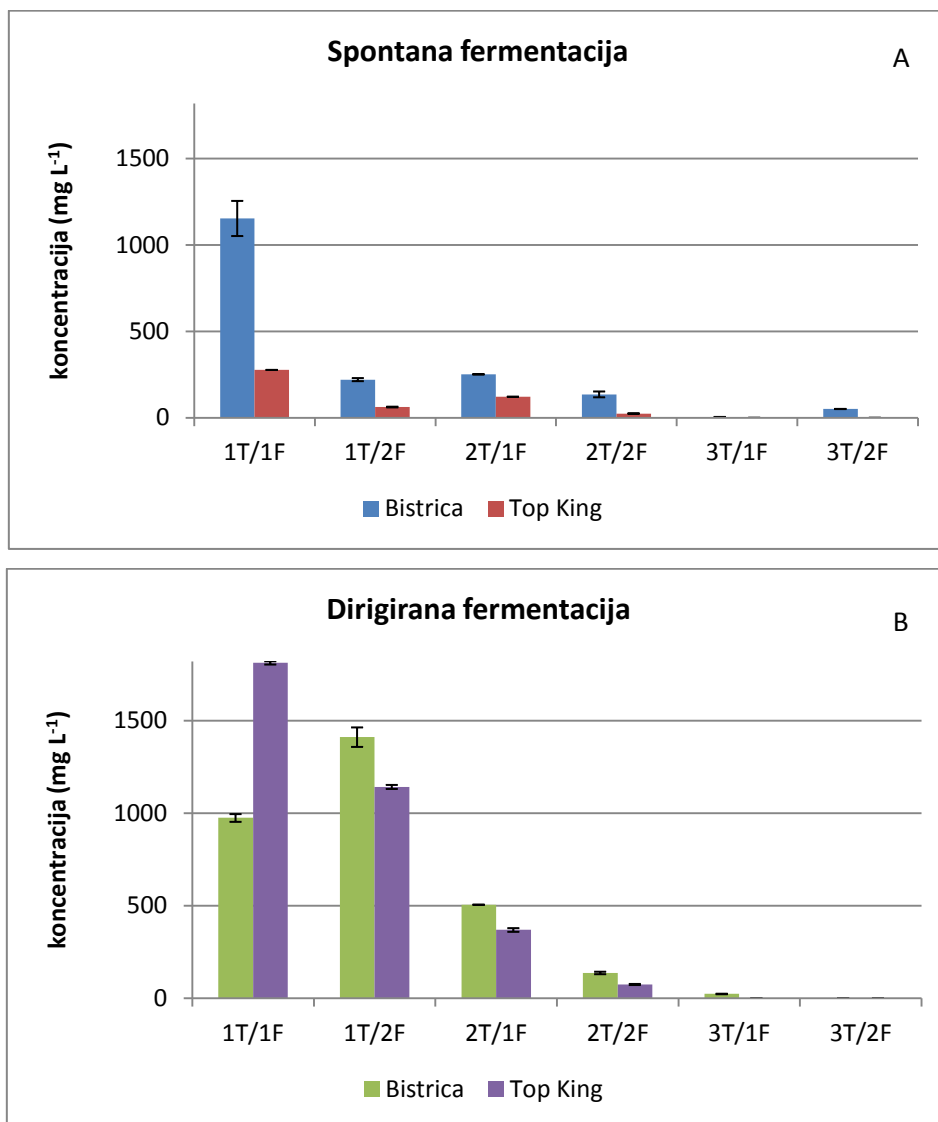
Slika 20. Usporedba koncentracija etil acetata u pojedinim frakcijama triju glavnih tokova destilata dobivenih destilacijom: A- spontano te B- dirigirano prefermentirane kominе šljive Bistrice i Top King.
