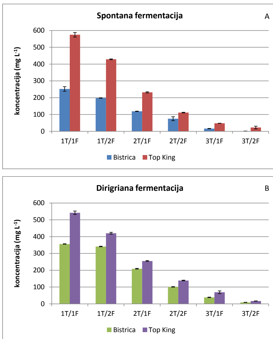
Slika 16. Usporedba koncentracija izobutanola u pojedinim frakcijama triju glavnih tokova destilata dobivenih destilacijom: A- spontano te B- dirigrano prefermentirane komine šljive Bistrice i Top King.
